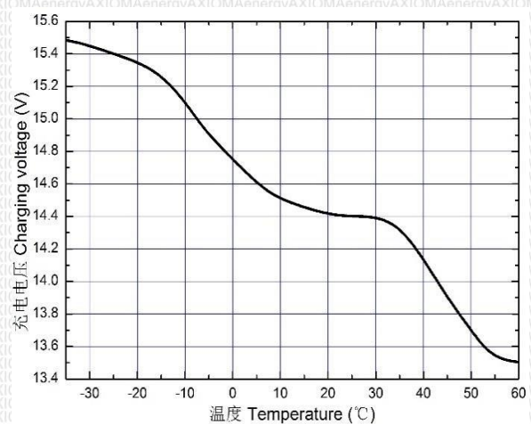
4 Зависимость зарядного напряжения от температуры
